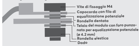
Dettagli del collegamento di terra:
